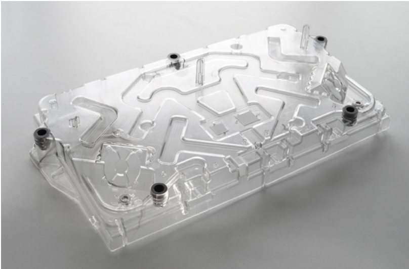
Abdeckung Klarglas Spritzguss mit Inserttechnik
