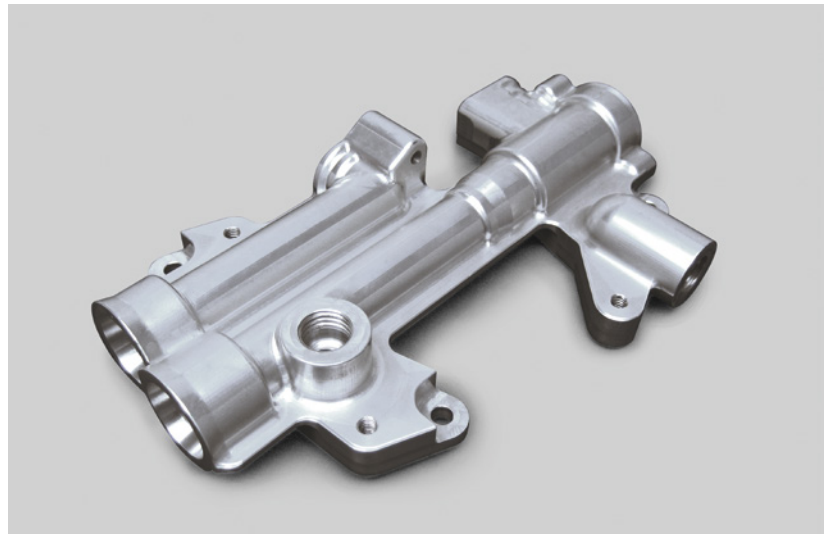
Verteiler 5-Achs-Bearbeitung
