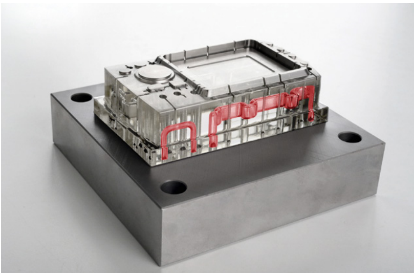
Einsatz Kamera (Visualisierung der konturnahen Kühlung) Lumex / Hybrid Additive Manufacturing
