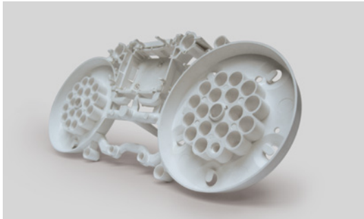
Lichtführung Spritzguss
